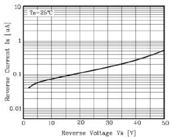
Fig. 2 I_R - V_R
