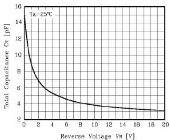
Fig. 3 C_T - V_R
